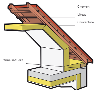
La continuité de l'isolation doit être assurée, en pied droit comme en rampant. La panne sablière doit aussi être isolée.
